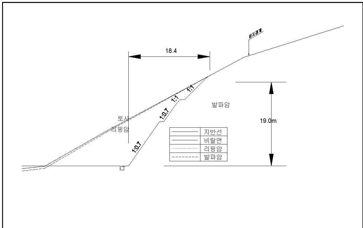
【안정검토 대표단면 산성휴게소(영천) Sta.0+530】
